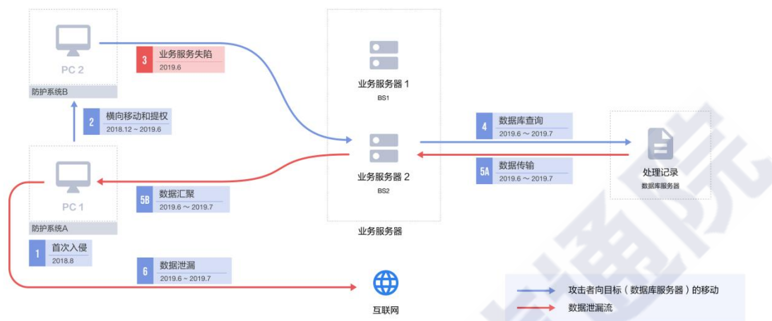
图 16 数据泄漏中的攻击移动和数据流
