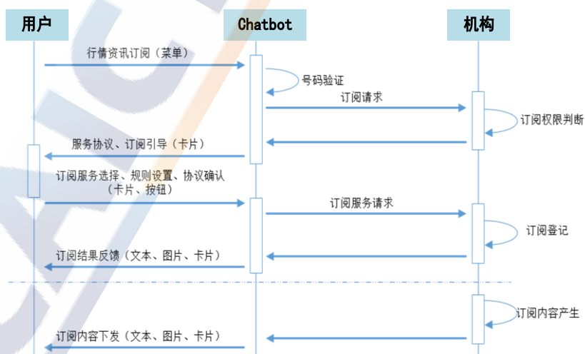
图 5 资讯订阅服务流程
